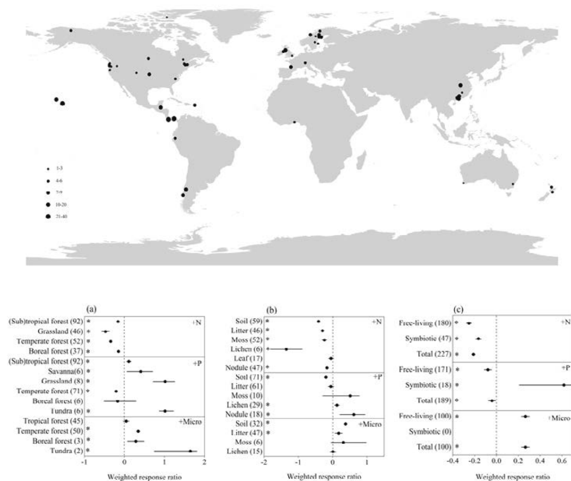
图. 养分添加对不同生态系统 (a)、固氮基质 (b) 和固氮类型 (c) 生物固氮的影响
