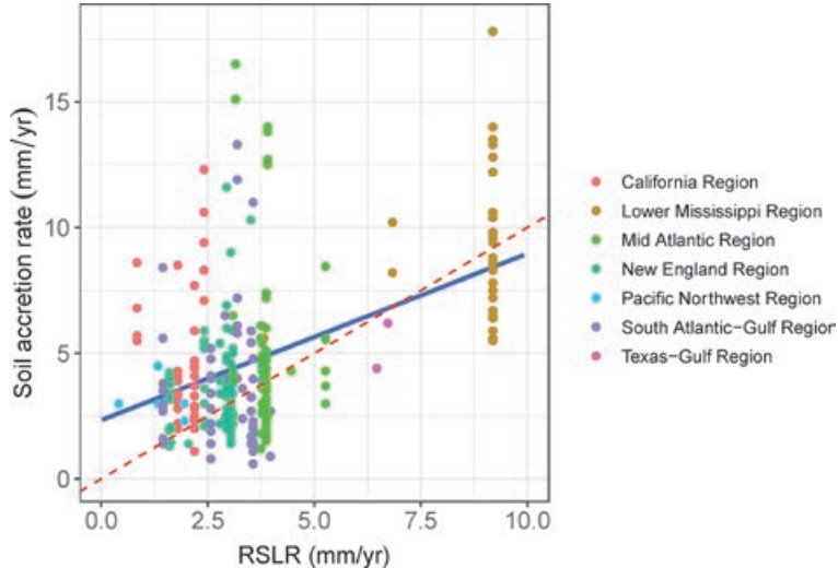
图 1. 海平面上升速率与滨海湿地沉积速率的比较
