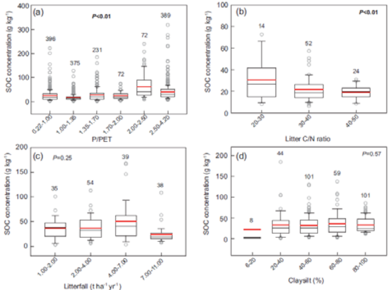
图 2. 基于已有文献数据分析得出的土壤有机碳 SOC (g C kg -1 ) 与 (a) 湿润指数 P/PET, (b) 凋落物 C/N, (c) 凋落物量 (t ha -1 yr -1 ), (d) 土壤粘粒 (%) 的相关关系
