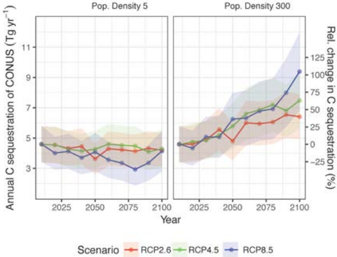
图 2. 未来不同气候变化情境下美国大陆滨海湿地年总固碳量的模型模拟结果
