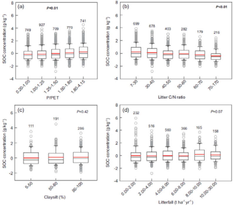
图 3. 基于中国森林生态系统调查和已发表数据分析得出的土壤有机碳 SOC (g C kg -1 ) 与 (a) 湿润指数 P/PET, (b) 凋落物 C/N, (c) 土壤粘粒 (%), (d) 凋落物量 (t ha -1 yr -1 ) 的相关关系
