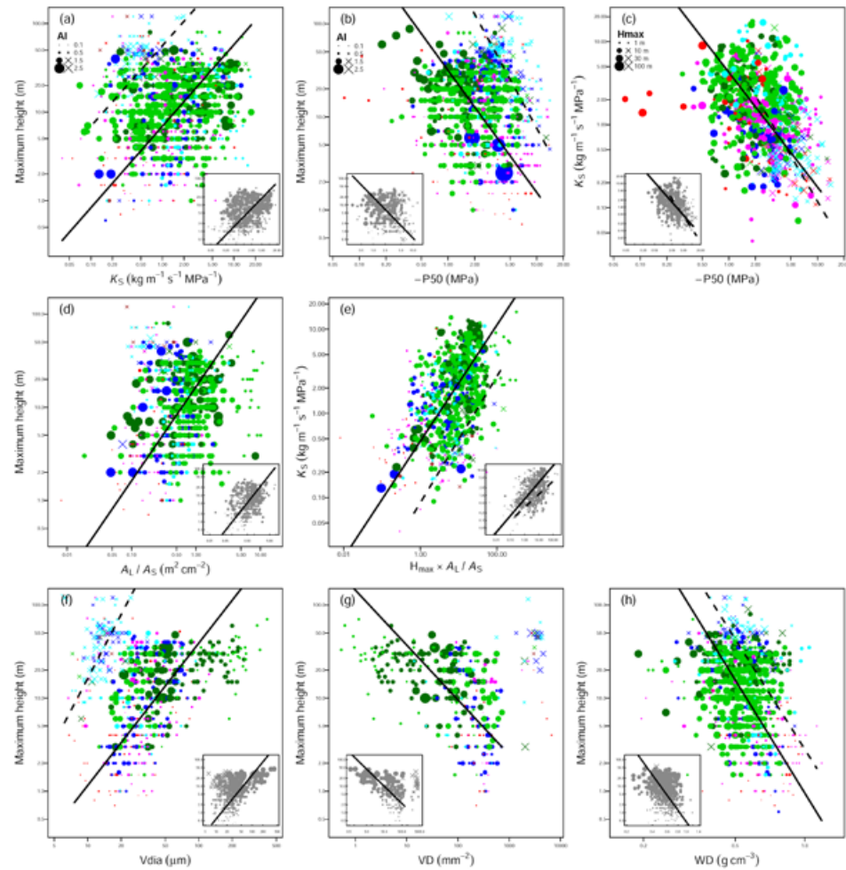
图 1. 全球尺度下植物水力性状与树高的协调关系。大图为最大树高，小图为实际树高；不同颜色代表不同生物区系；圆点实线为被子植物，叉和虚线为裸子植物。用以分析的水力性状为 (a) 木质部枝条比导水率 (Ks); (b) 水力导度损失 50% 的木质部水势 (P50); (c) Ks 和 P50 的权衡关系; (d) 叶边材面积比 (AL/AS); (e) 验证达西定律; (f) 导管 / 管胞直径 (Vdia); (g) 导管 / 管胞密度 (VD); (h) 边材密度 (WD)
